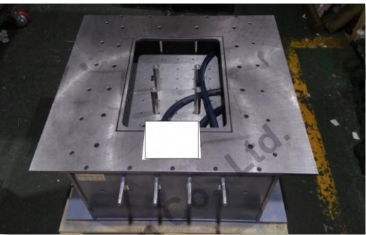
중대형 금형/가공품(냉각모듈)
