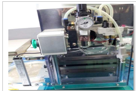
동판 프레스 02
